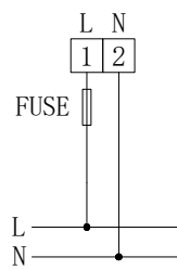
AMB1X0-A(W)-P1 辅助电源
