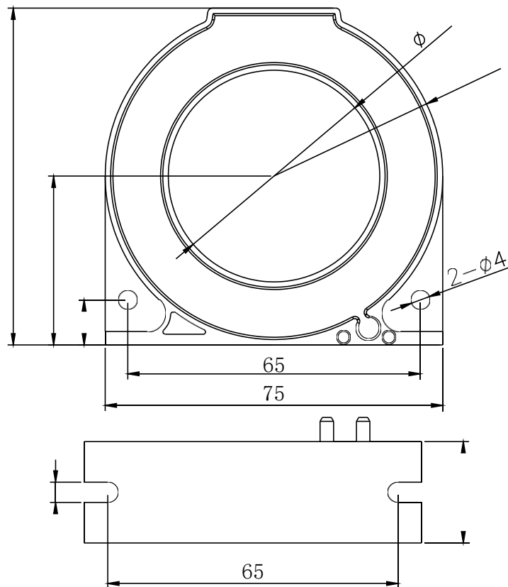
AKH-0.66/W-45NY 系列互感器
